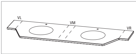
APD 809V_(Grundkörper 1.800 mm) APN 80VR_(Verlängerung Rechts) APN 80VL_(Verlängerung Links) APN 80VM_(Verlängerung Mitte)
