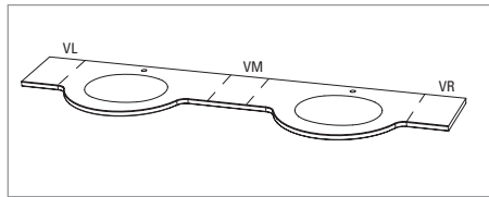
APD 819V_(Grundkörper 1.800 mm) APN 81VR_(Verlängerung Rechts) APN 81VL_(Verlängerung Links) APN 81VM_(Verlängerung Mitte)
